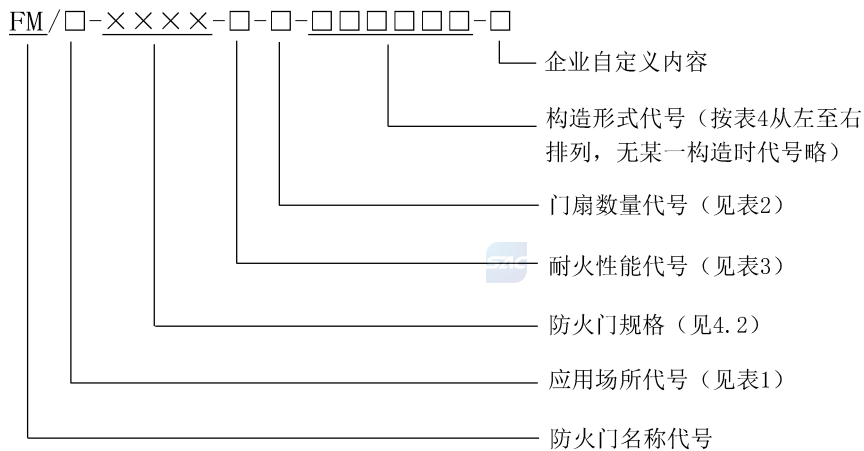
图 1 防火门型号编制
